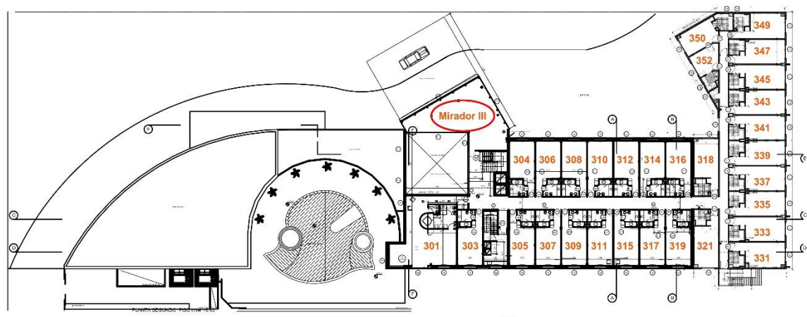
PLANTA SEGUNDO PISO nivel +8.40 - 30 HABITACIONES Escala 1:100
