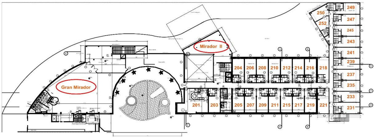
PLANTA NIVEL 2 - PRIMER PISO +30 HABITACIONES
